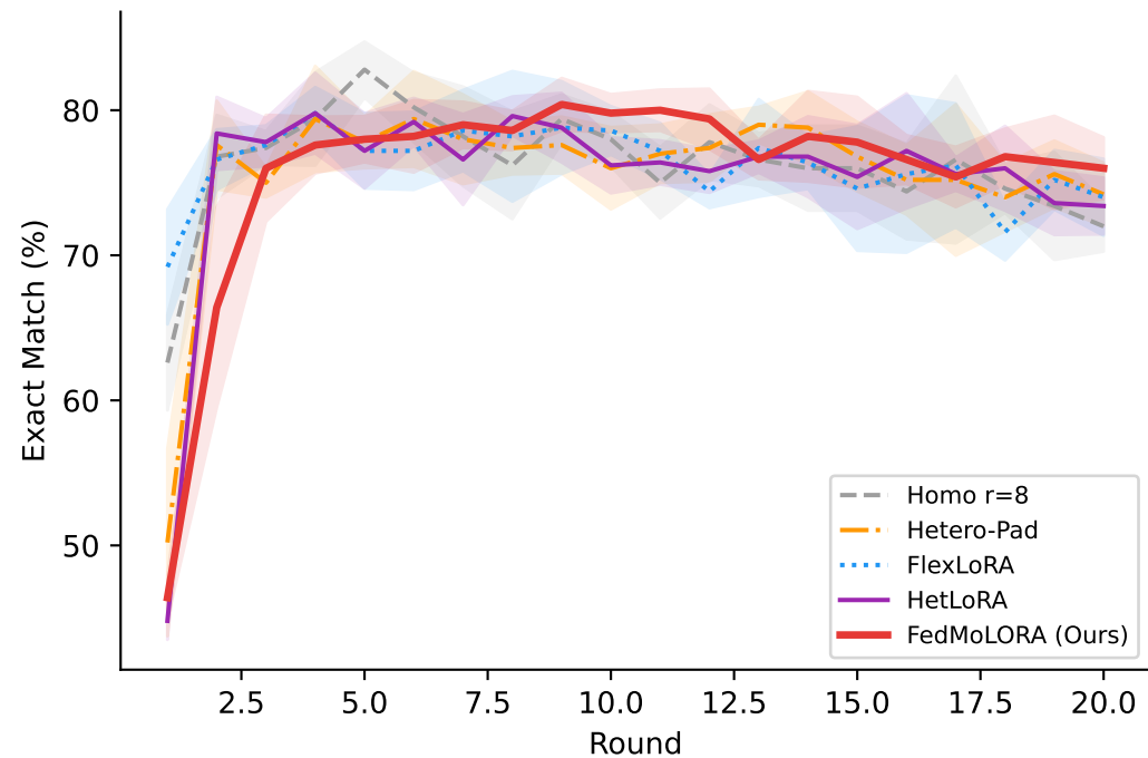
GSM8K \alpha=0.5
