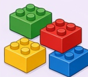
Lego
