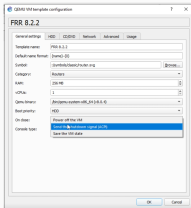
Рис. 26: ACPI
