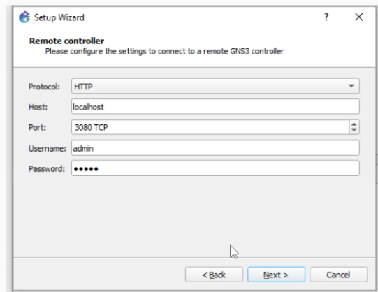
Рис. 14: Подключение
