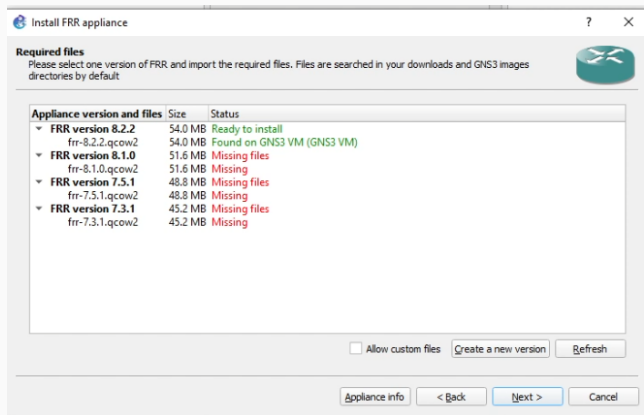
Рис. 22: Успешный импорт
