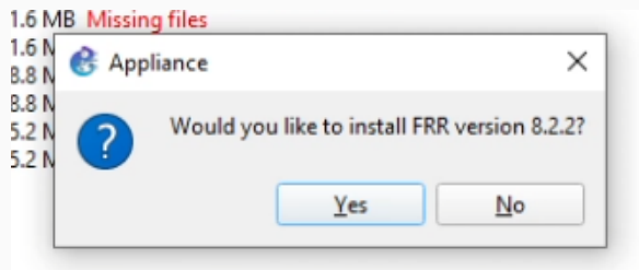
Рис. 23: Соглашение
