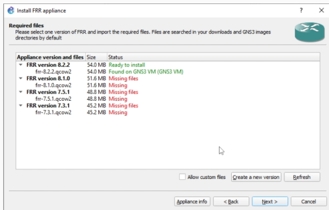
Рис. 20: Скачивание образа
