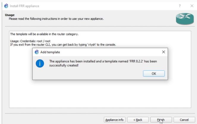
Рис. 24: Успешная установка
