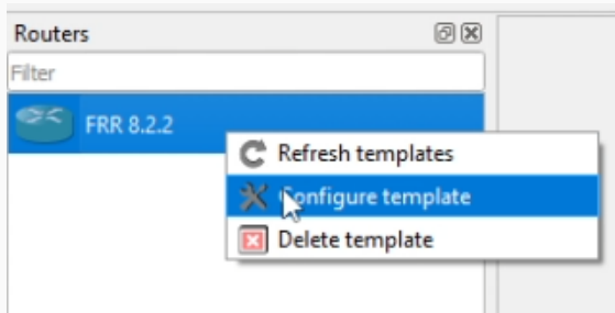
Рис. 25: Конфигурация темплейта
