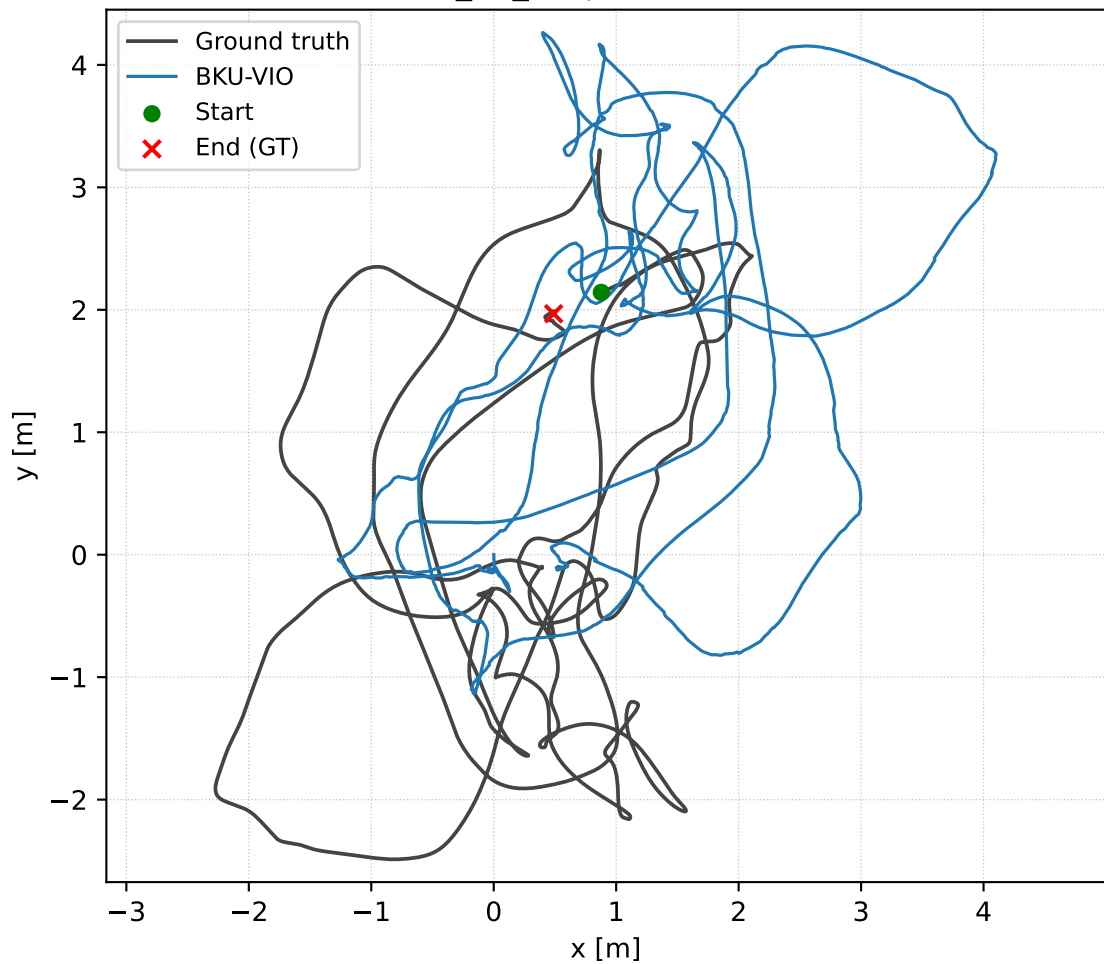
EuRoC V1_01_easy - BKU-VIO baseline
