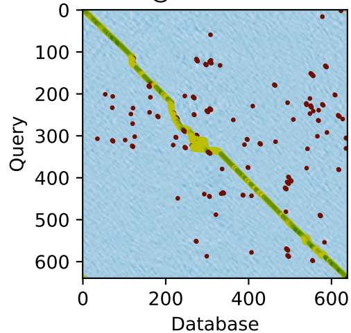
R@1 = 0.7063
