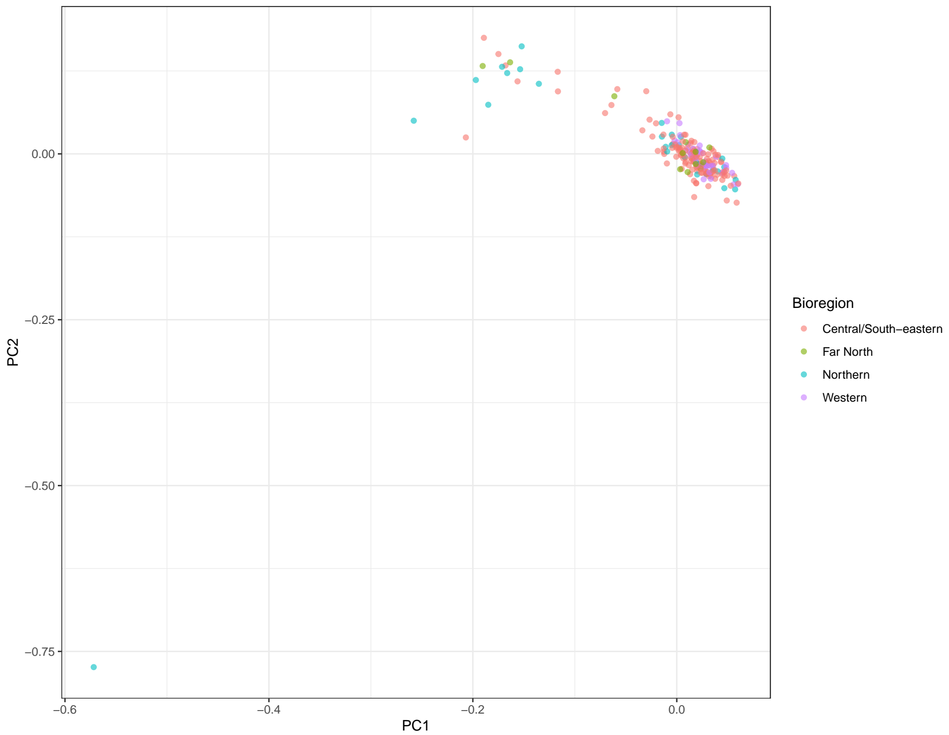
Local PCA – Chromosome 6
