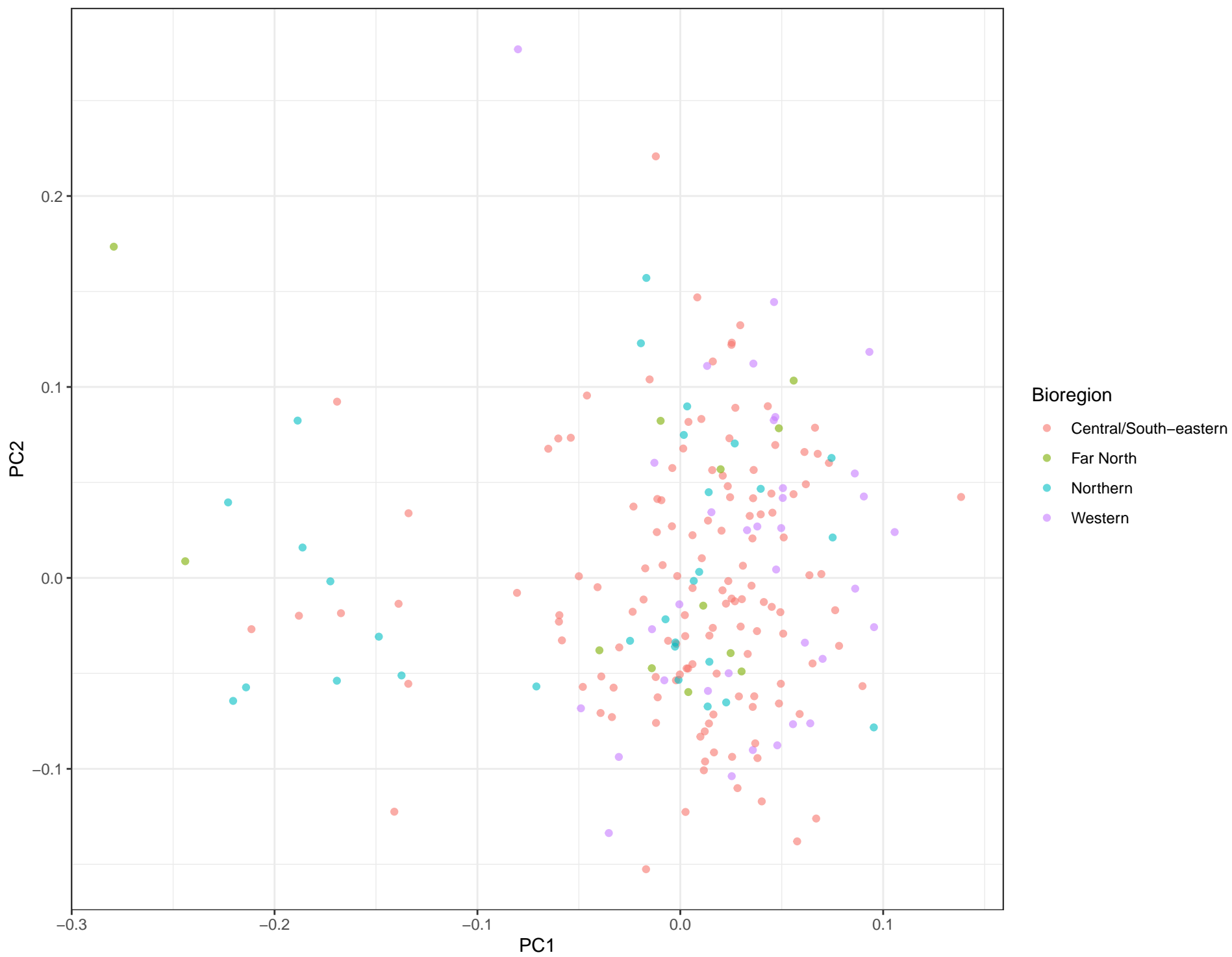
Local PCA – Chromosome 5
