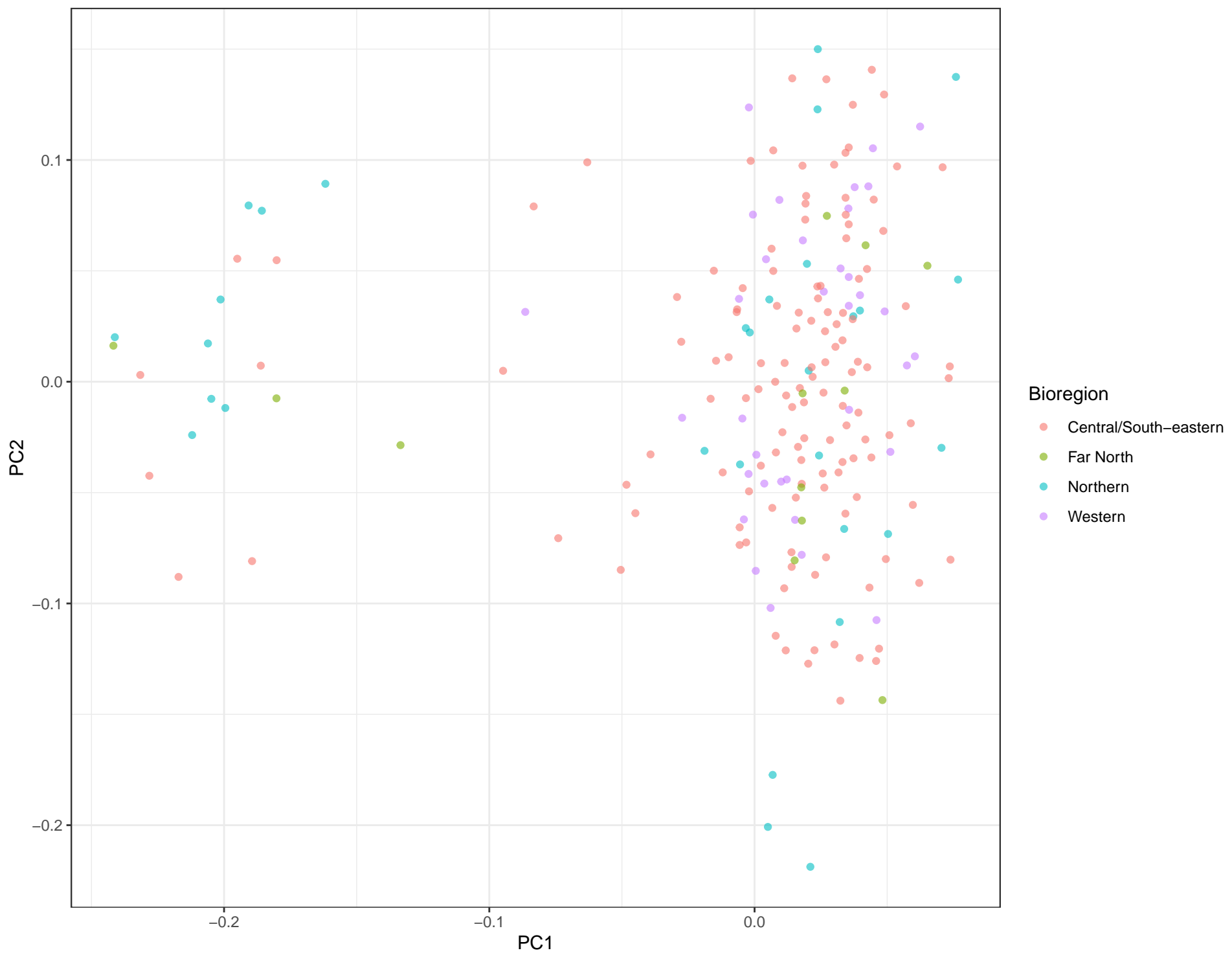
Local PCA – Chromosome 19
