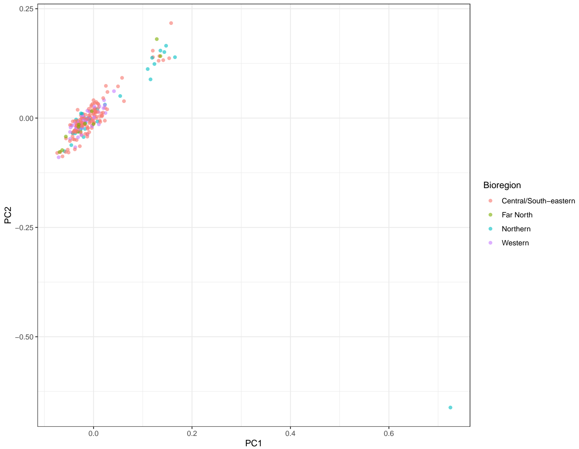
Local PCA – Chromosome 12
