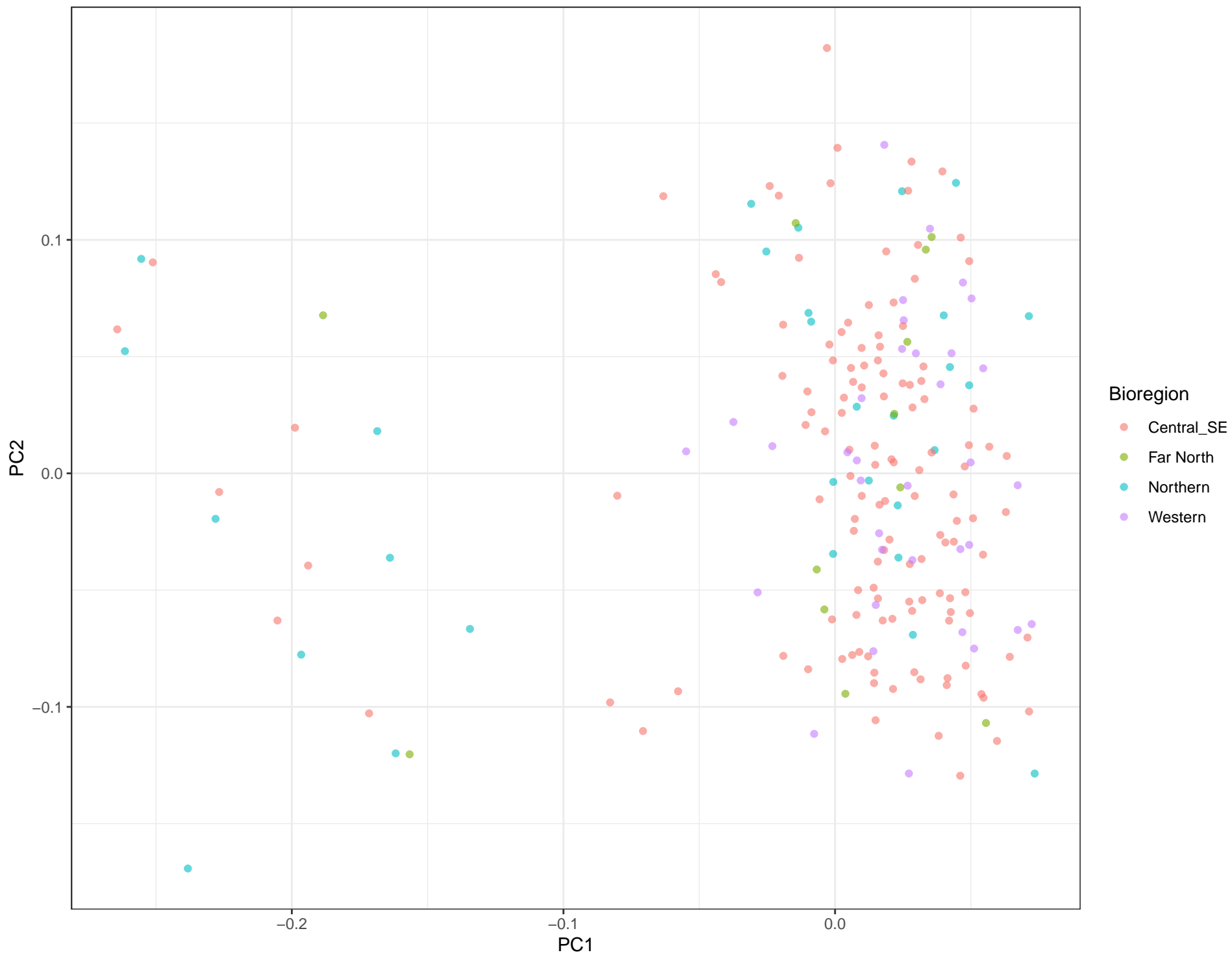
Local PCA – Chromosome 2
