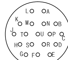
YH3474W14-18SN연결 기 후면도 #20-18EA
