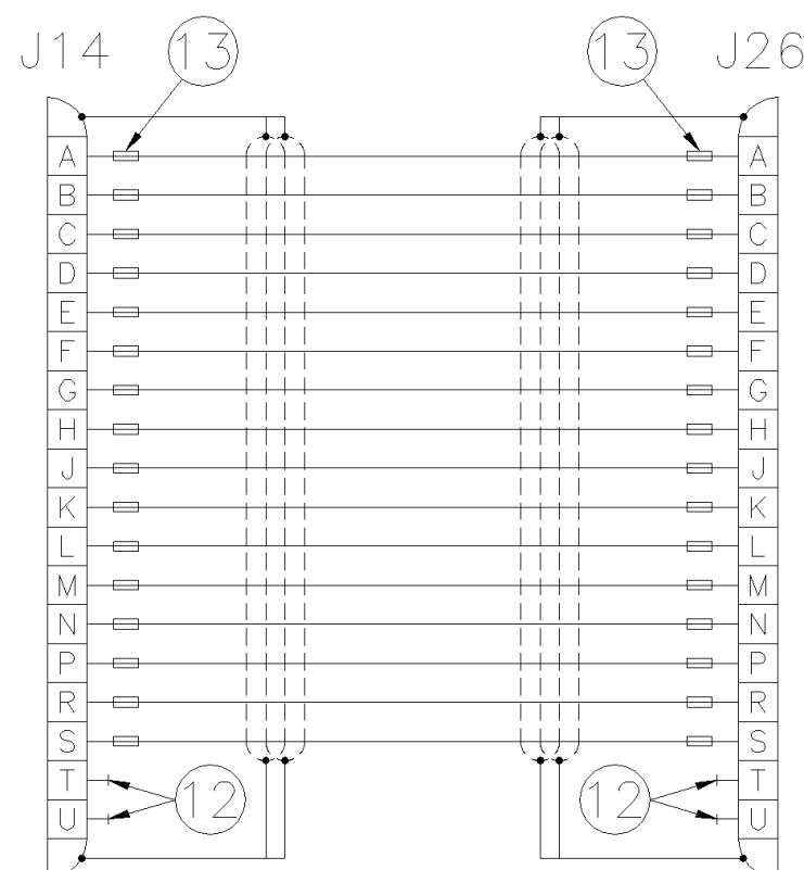
음성 및 전원 공급기 0A-7086K-J14와 연결
