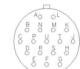
MS3475 W14-18P (18개 20콘택트)
