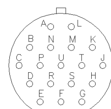
MS3475 W14-18P (18개 20콘택트)
