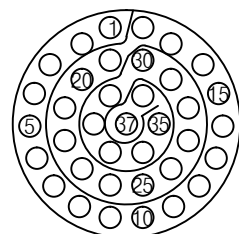
YH38999/26FD35PN 연결기 후면도 #22D-37EA
