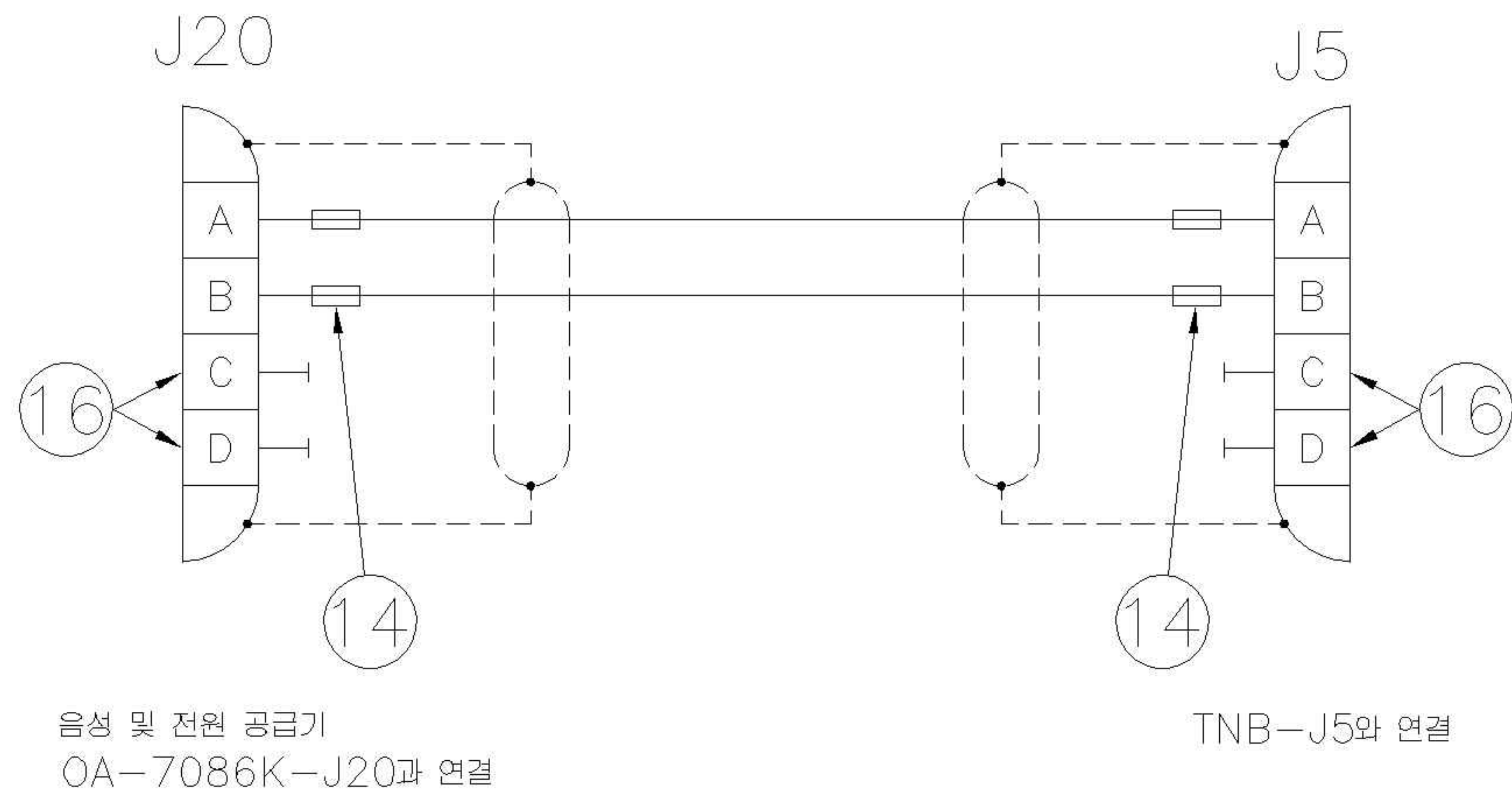
케 이 블 결 선 도
