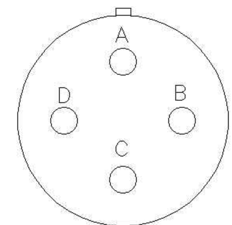
OA-7086K-J20 (4개 12콘택트)
