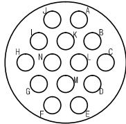
YH3100A20-27SN 연결기 후면도 #16-14EA
