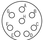
YH3100A20-7SN 연결기 후면도 #16-8EA
