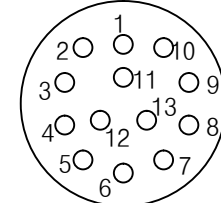
YH38999/44FB35PN 연결기 후면도 #22D-13EA
