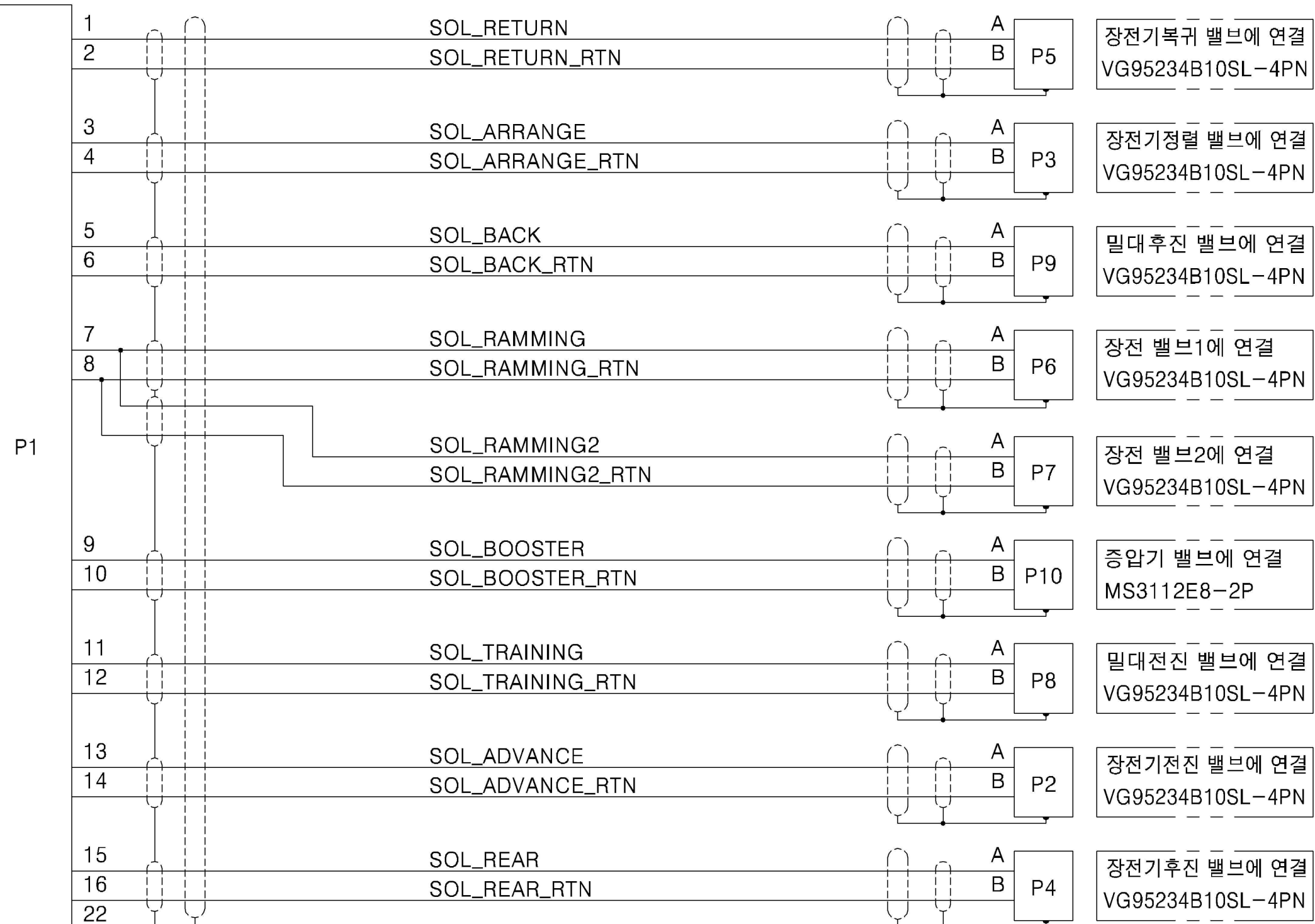
회로도
