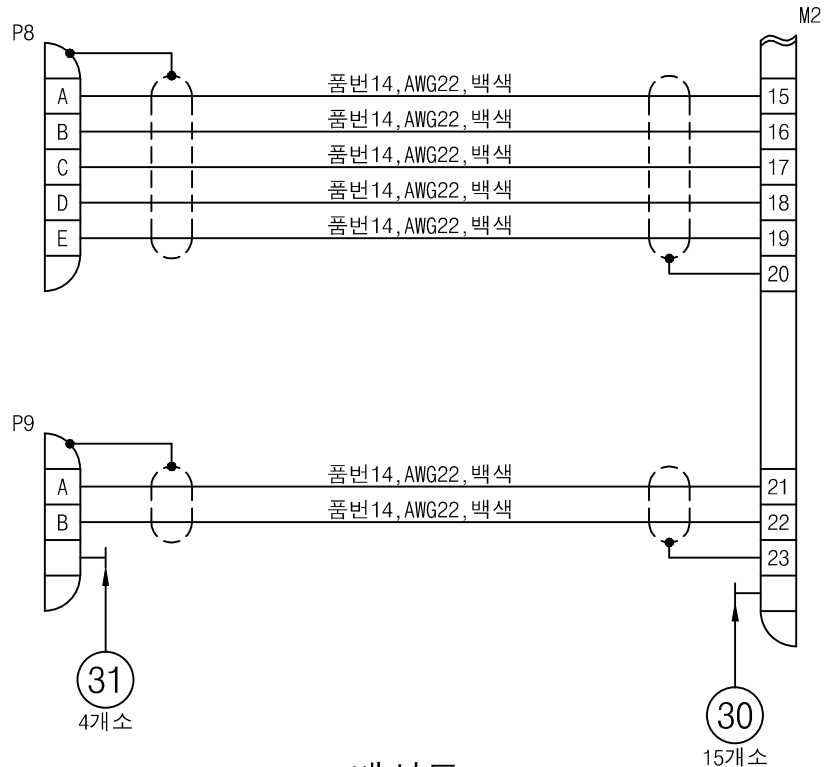
배선도
