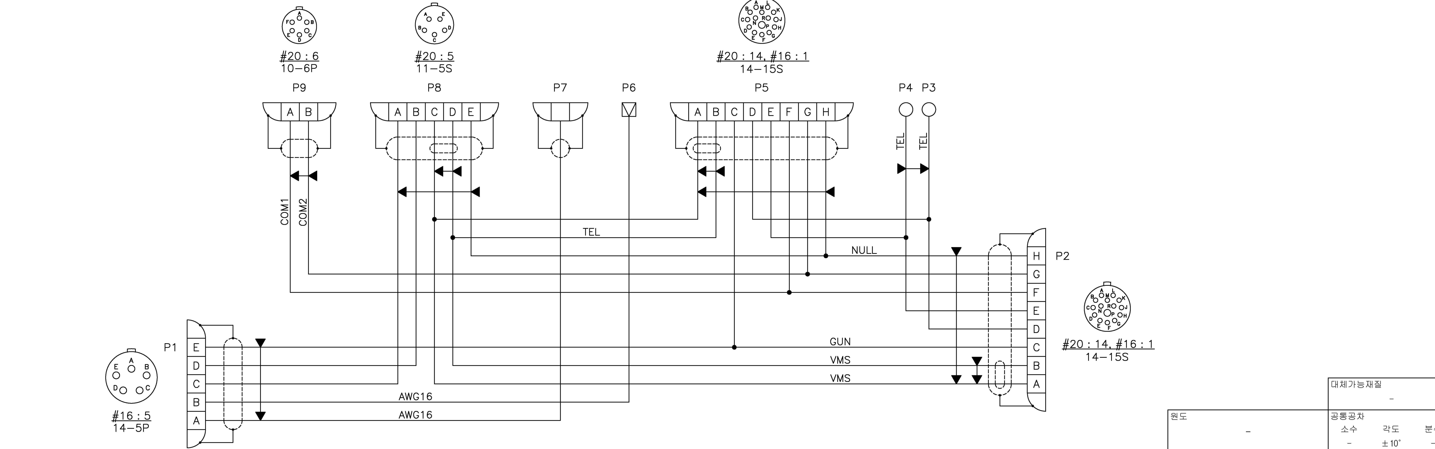
배선도
