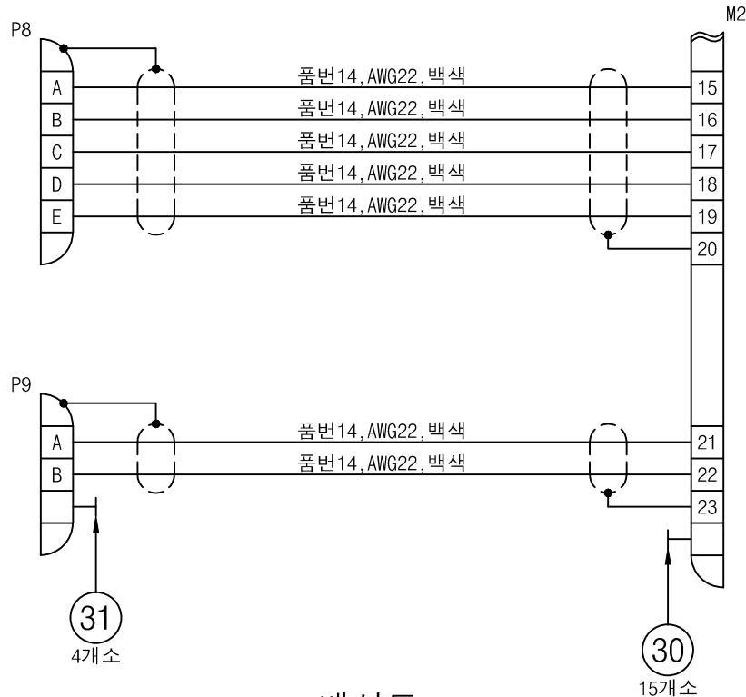
배선도
