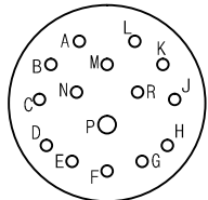
YH3475W14-15PN 연결기 후면도 #20-14EA #16-1EA
