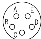
YH27468T11F5PN 연결기 후면도 #20-5EA
