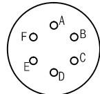
YH3474W10-6SN 연결기 후면도 #20-6EA
