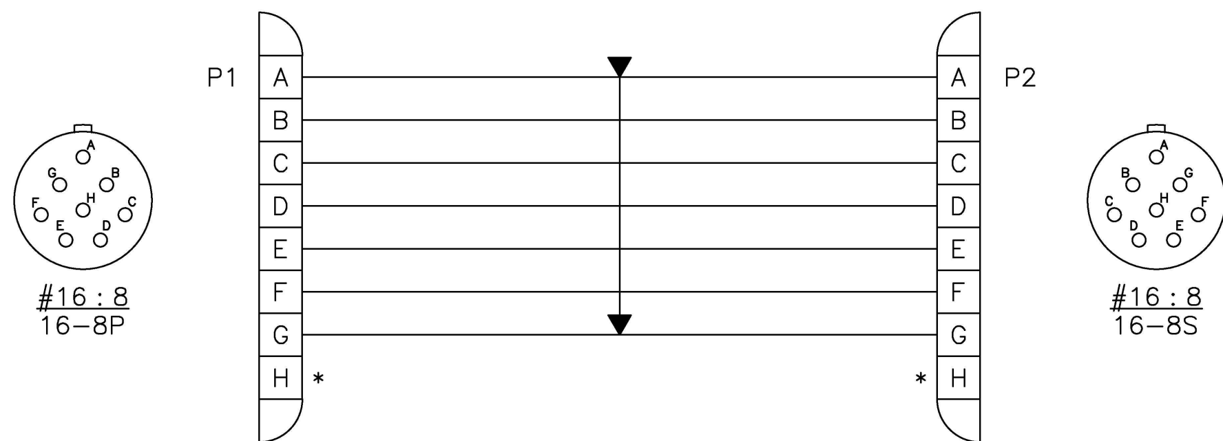
배선도
