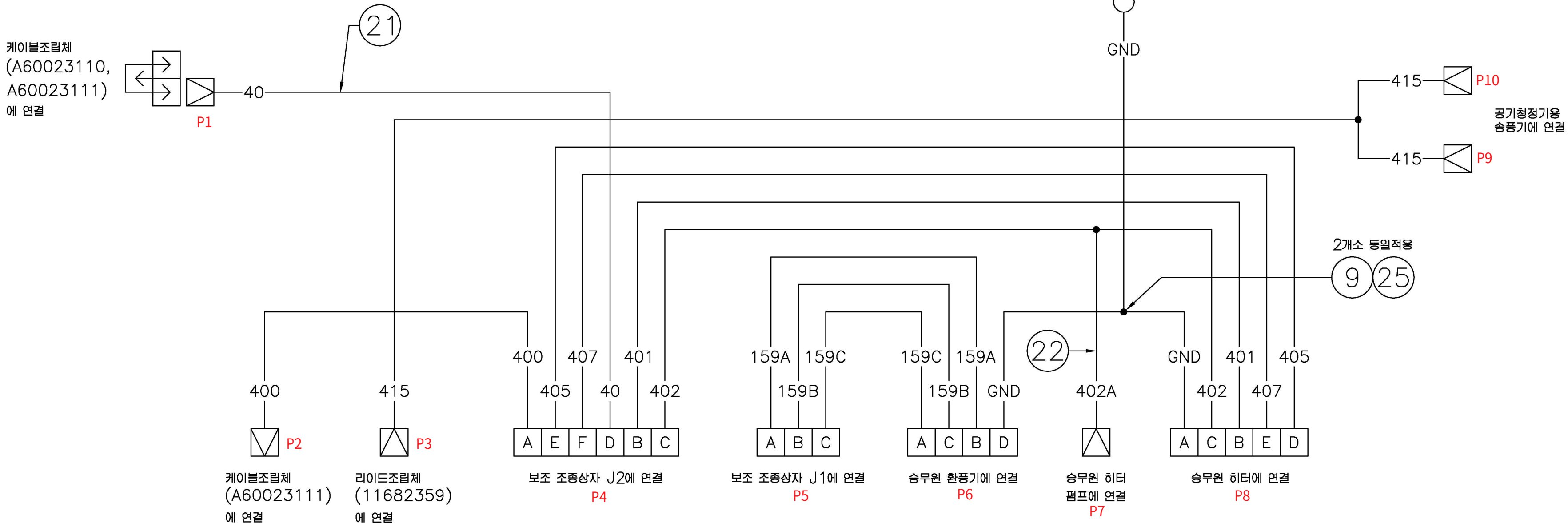
배선도
