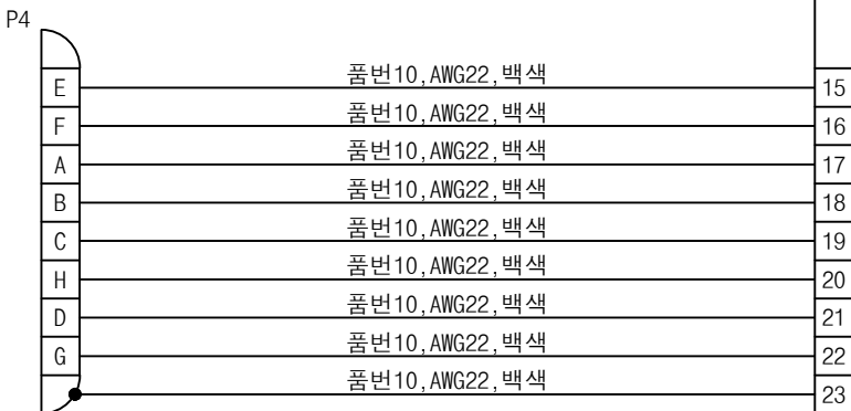
YH3100A22-23PN 연결기 후면도 #12-8EA
