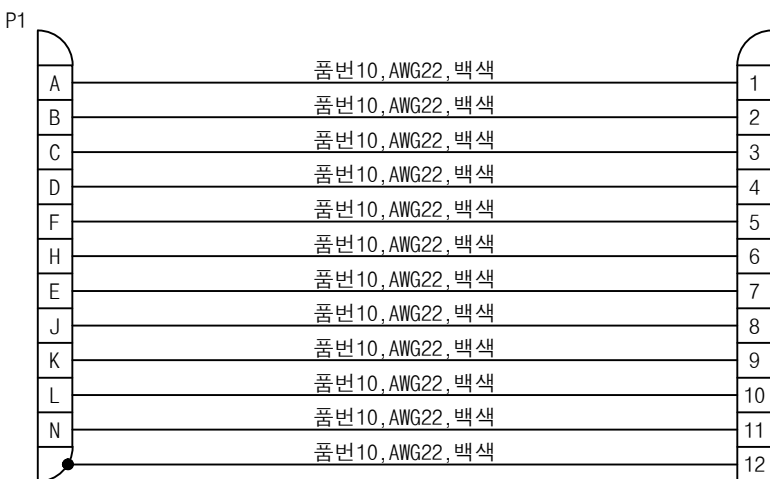
YH3100A28-51PN 연결기 후면도 #12-12EA
