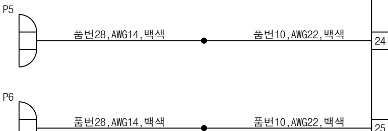
MS27142-2 연결기 후면도 #14-1EA
