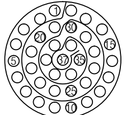
YH38999/26FD35PN 연결기 후면도 #22D-37EA
