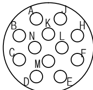
YH3100A28-51PN 연결기 후면도 #12-12EA
