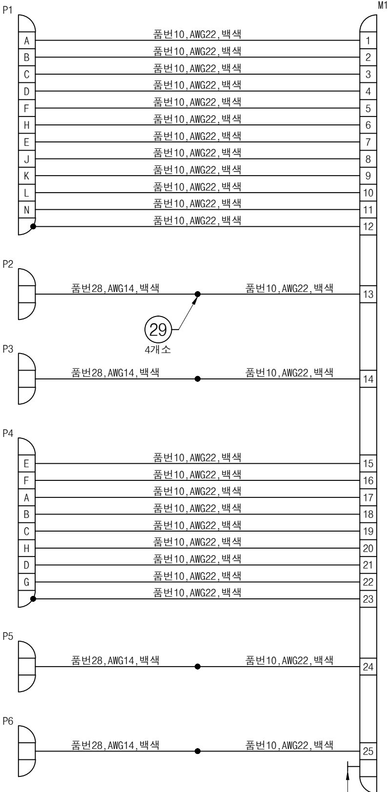
배선도
