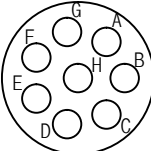
YH3100A22-23PN 연결기 후면도 #12-8EA
