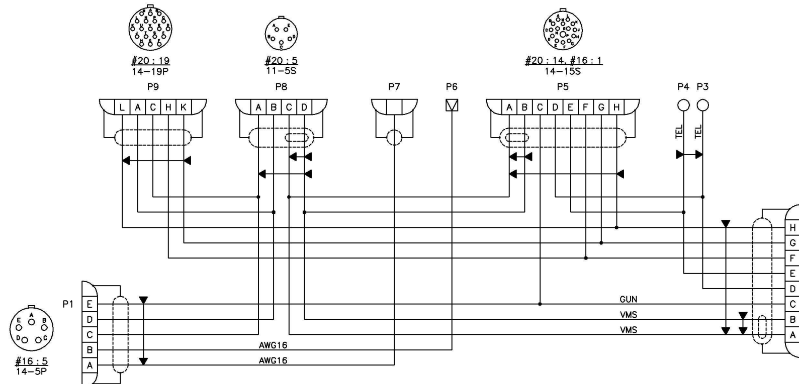
배선도
