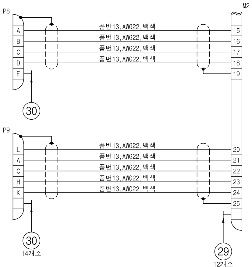
배선도
