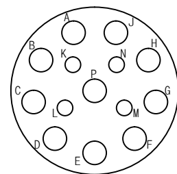
YH3100A28-20PN 연결기 후면도 #16-4EA #12-10EA
