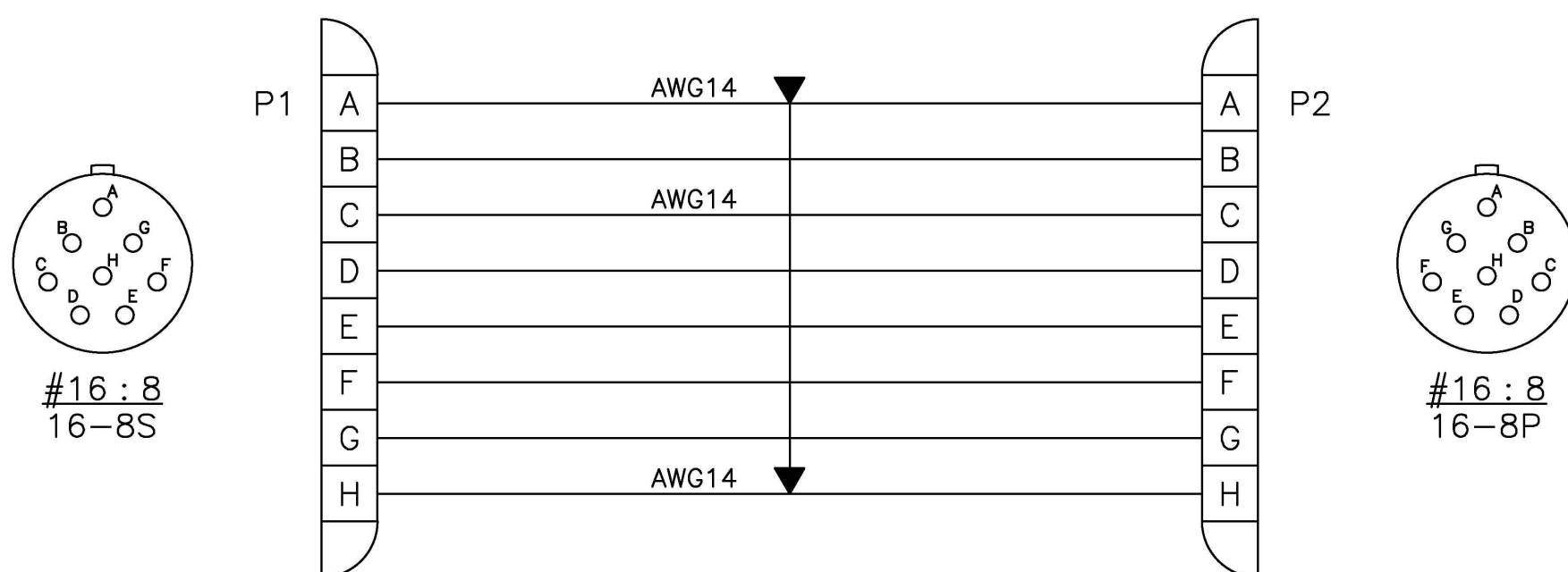
배선도
