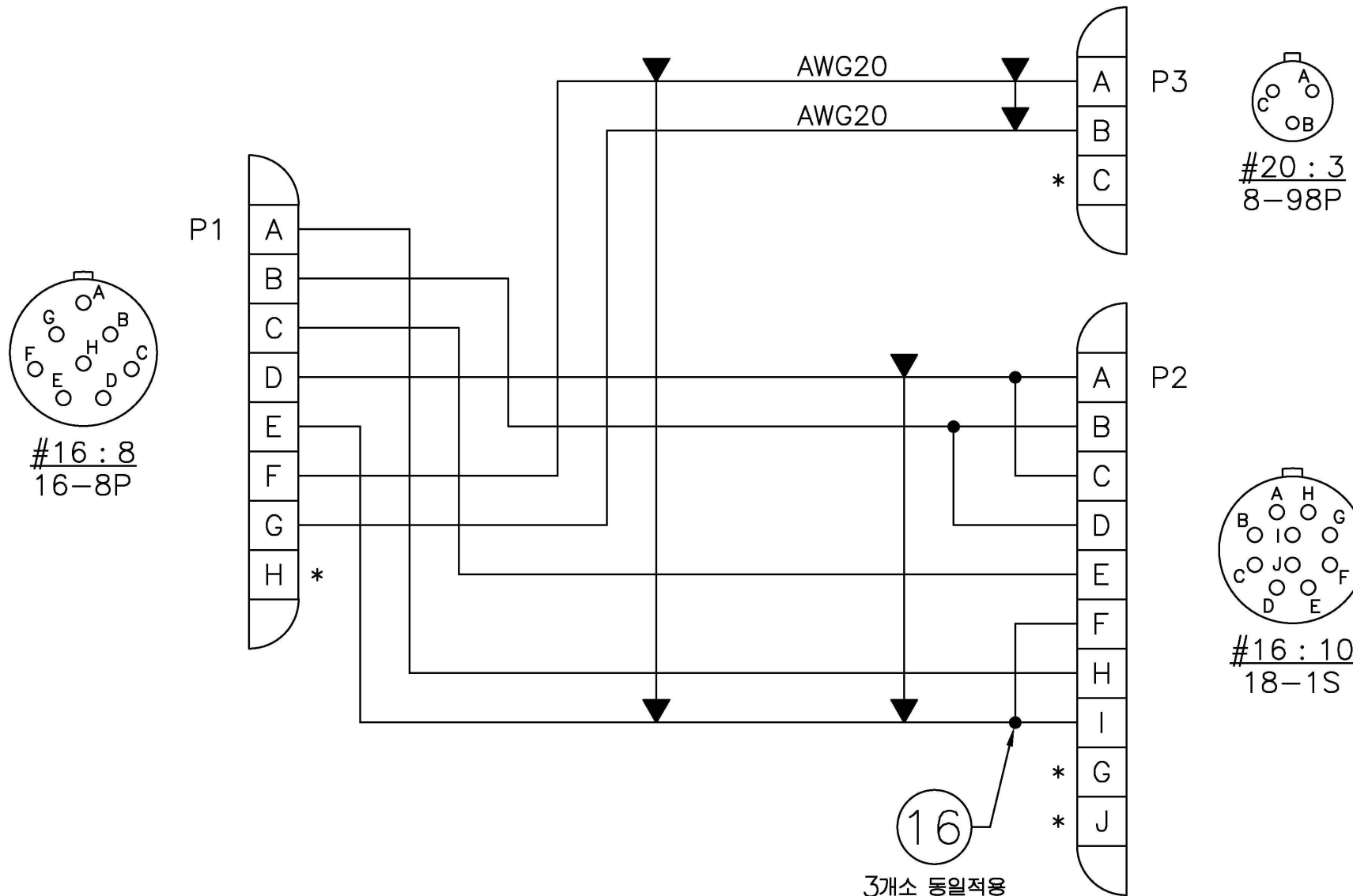
배선도
