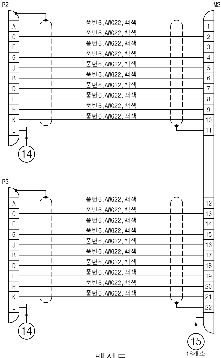
배선도
