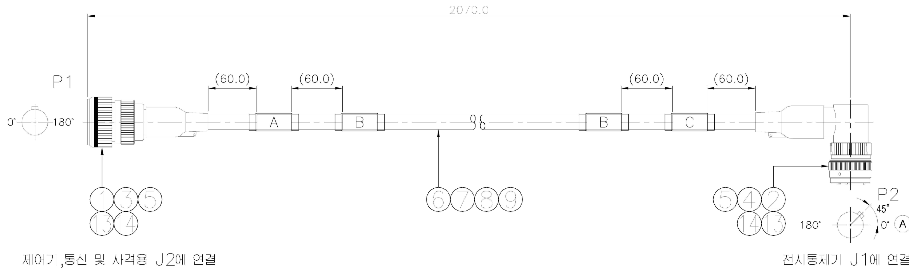
케이블 결선도
