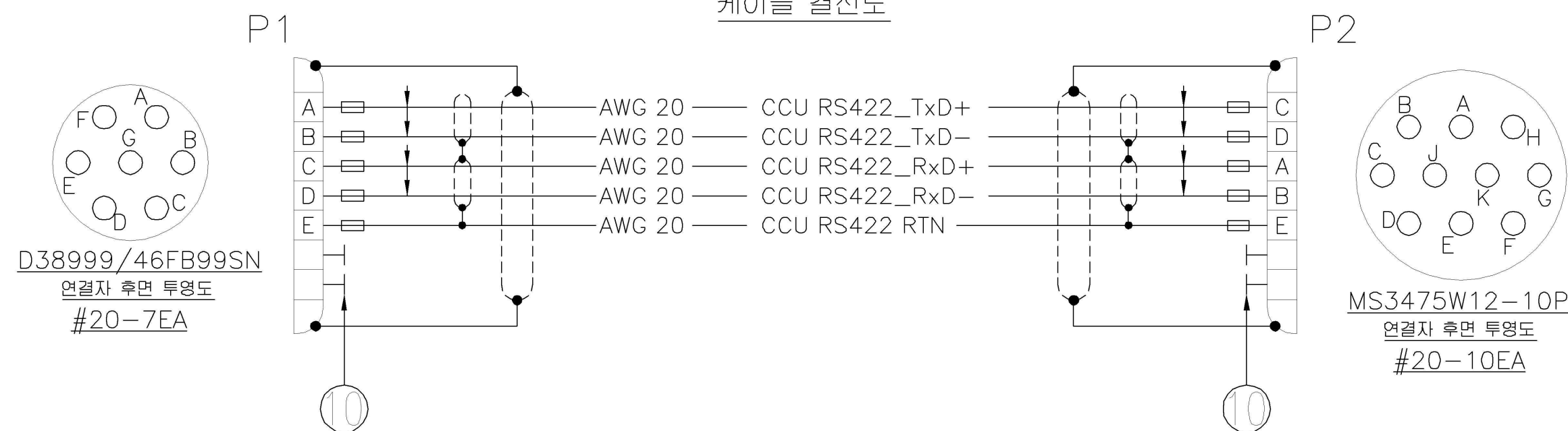
케이블 결선도
