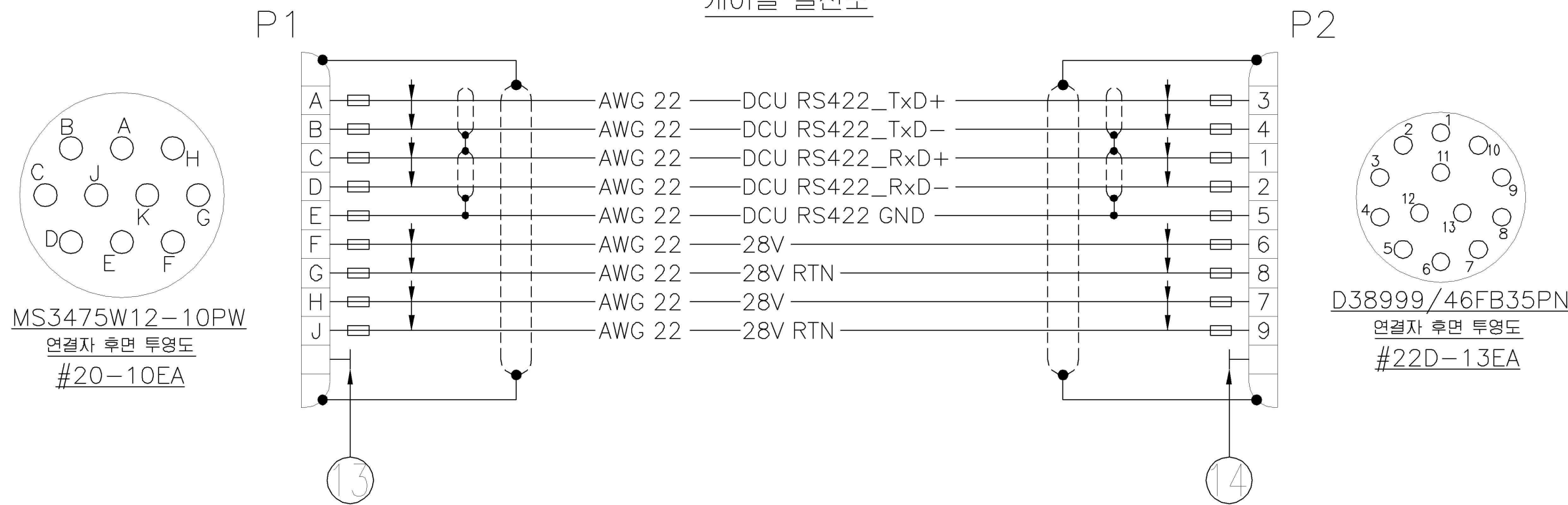
케이블 결선도
