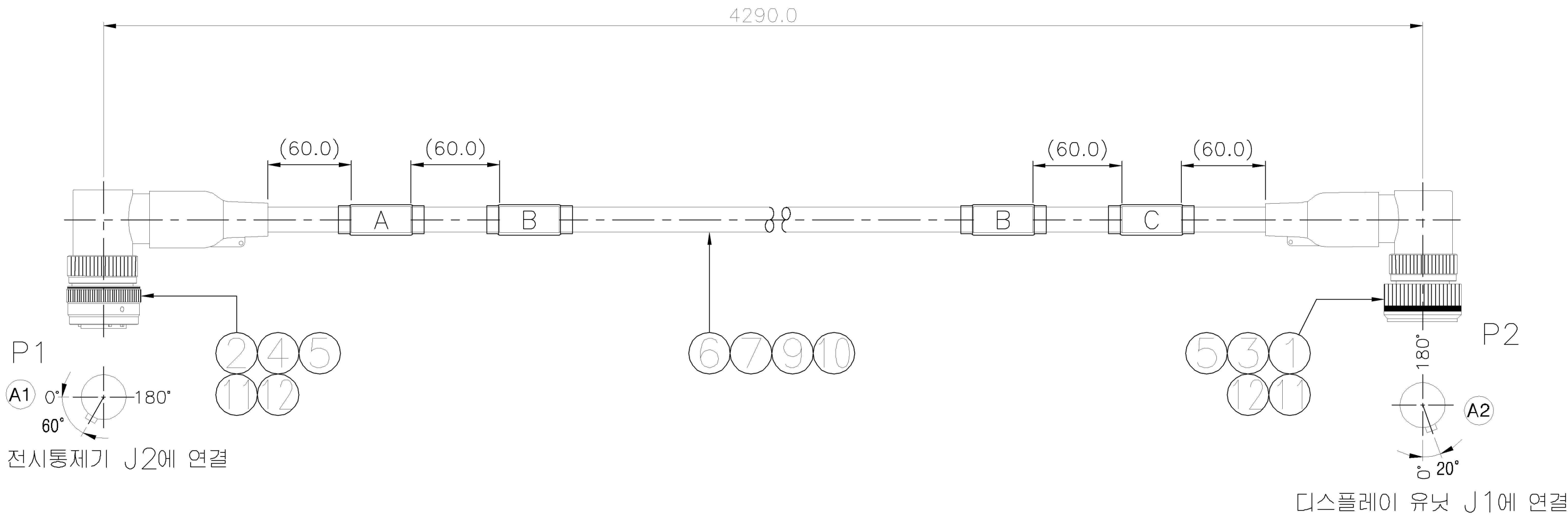
케이블 결선도
