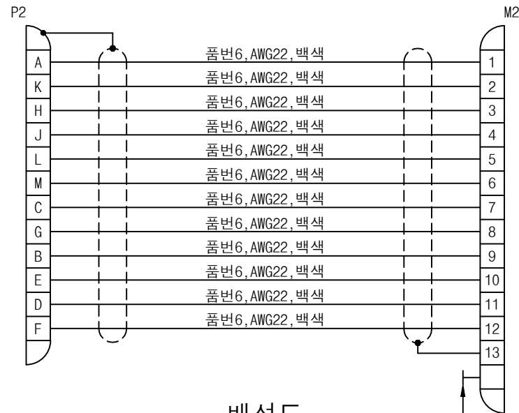
배선도
