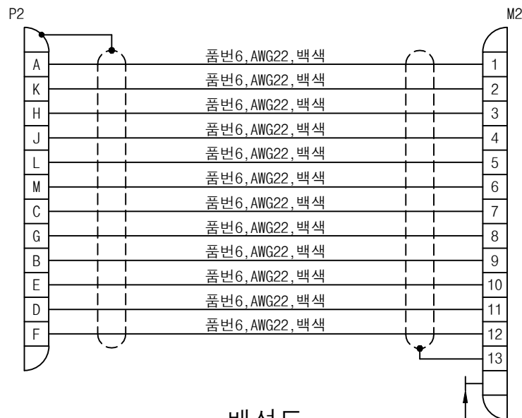
배선도
