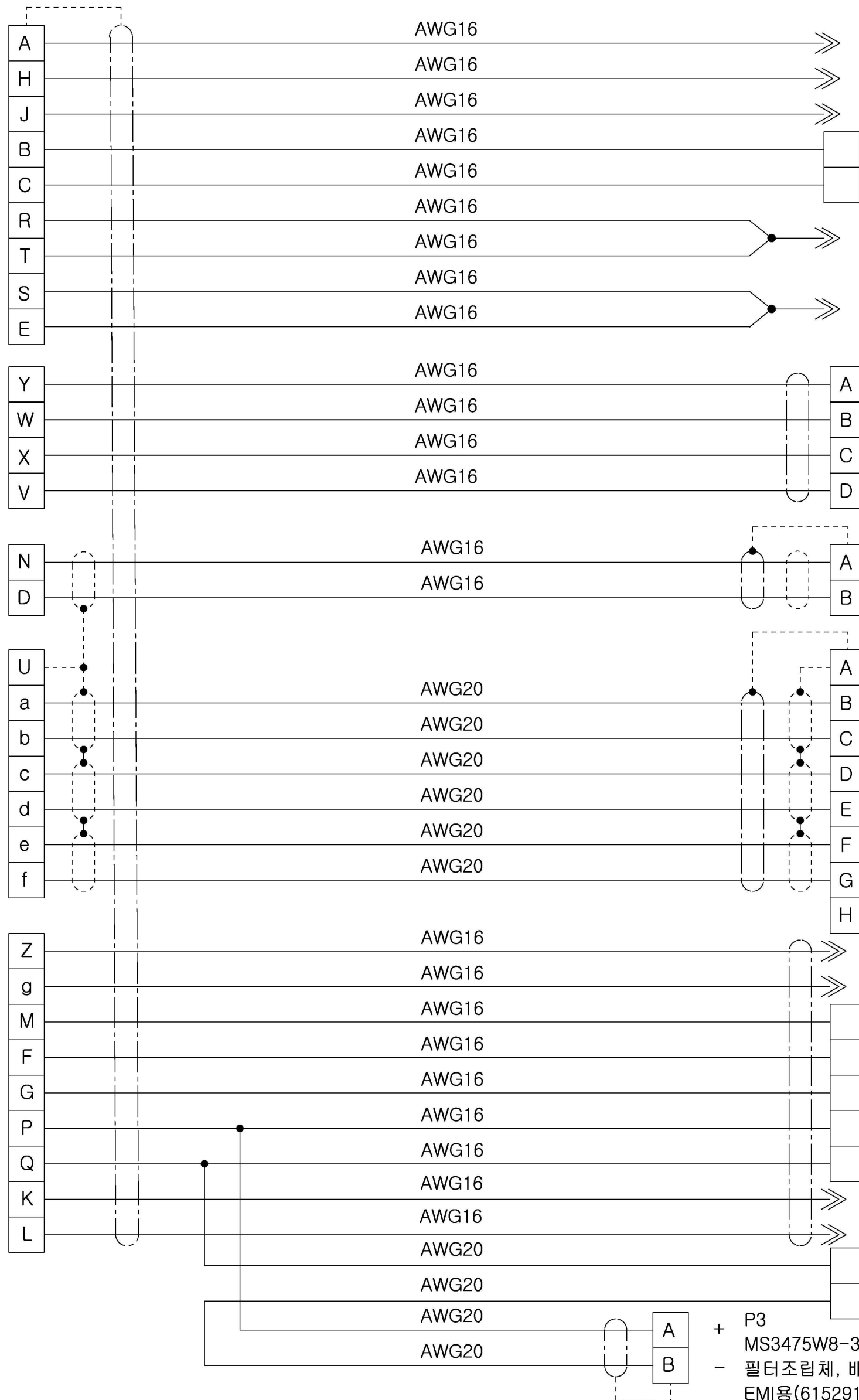
배선도
