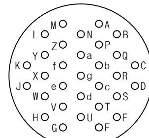
YH3474W24-31SN연결 기 후면도 #16-31EA
