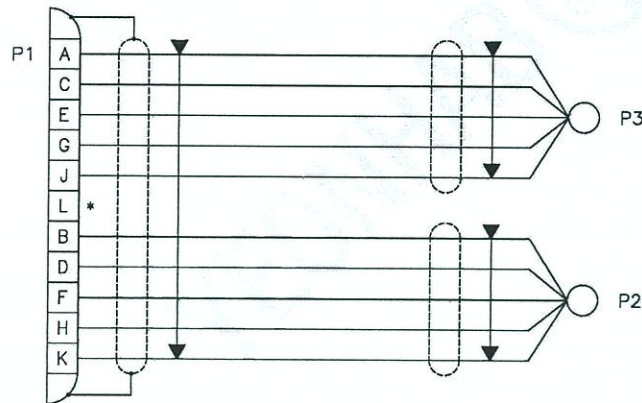
배선도
