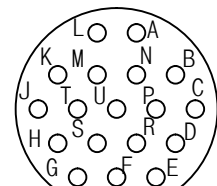
YH27468T15F18SN 연결기 후면도 #20-18EA
