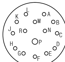
YH3474W14-15SN 연결기 후면도 #16-1EA #20-14EA
