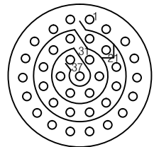
YH38999/44FD35SA 연결기 후면도 #22D-37EA
