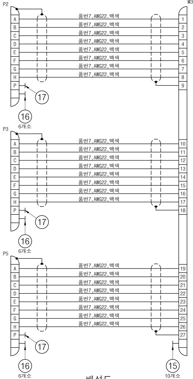
배선도
