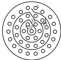
YH38999/44FD35SA 연결기 후면도 #22D-37EA
