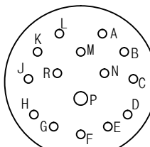
YH3474W14-15SN 연결기 후면도 #16-1EA #20-14EA
