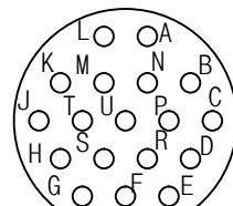
YH27468T15F18SN 연결기 후면도 #20-18EA
