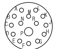
YH38999/24WD15PN 연결기 후면도 #20-14EA #16-1EA
