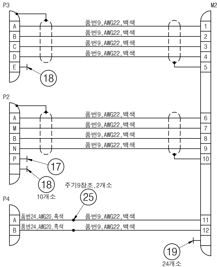
배선도
