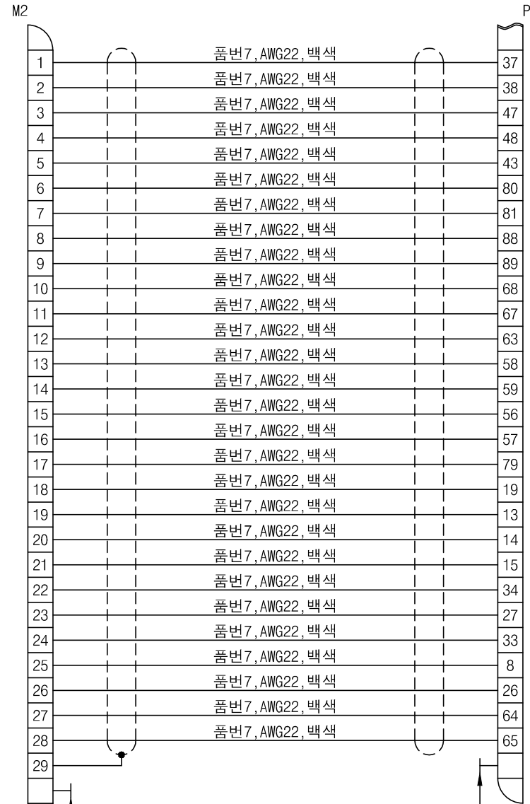
배선도
