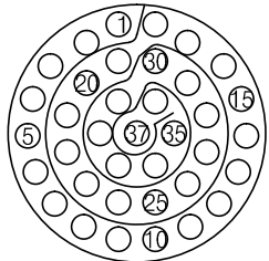
YH38999/26FD35PN 연결기 후면도 #22D-37EA
