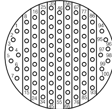
YH38999/24WH35PN연 결기 후면도 #22D-100EA
