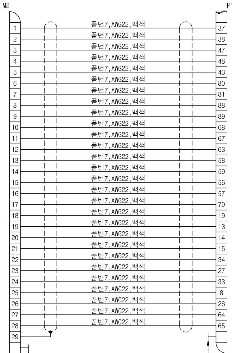
배선도
