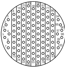
YH38999/24WH35PN연 결기 후면도 #22D-100EA
