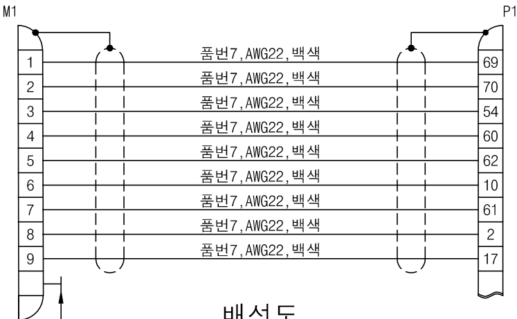
배선도
