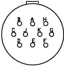
C : 표 참조 (10개 20콘택트)
