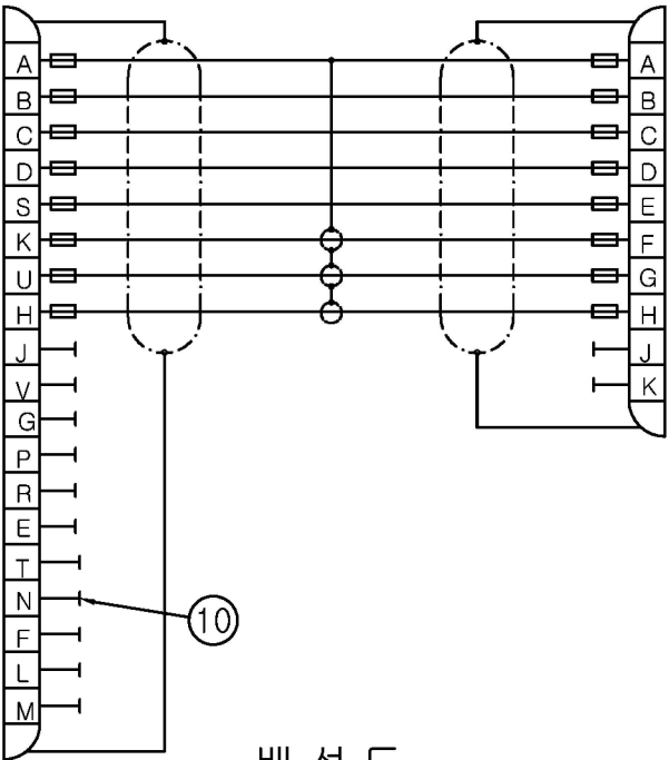
배 선 도
