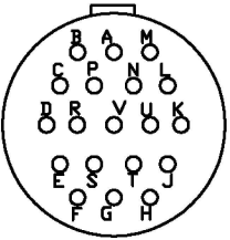
B : 표 참조 (19개 20콘택트)
