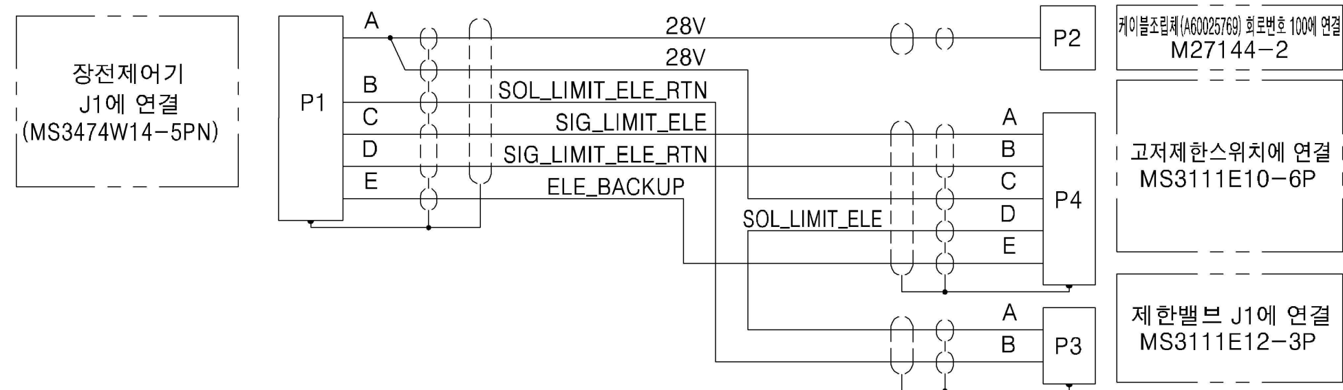
회로도
