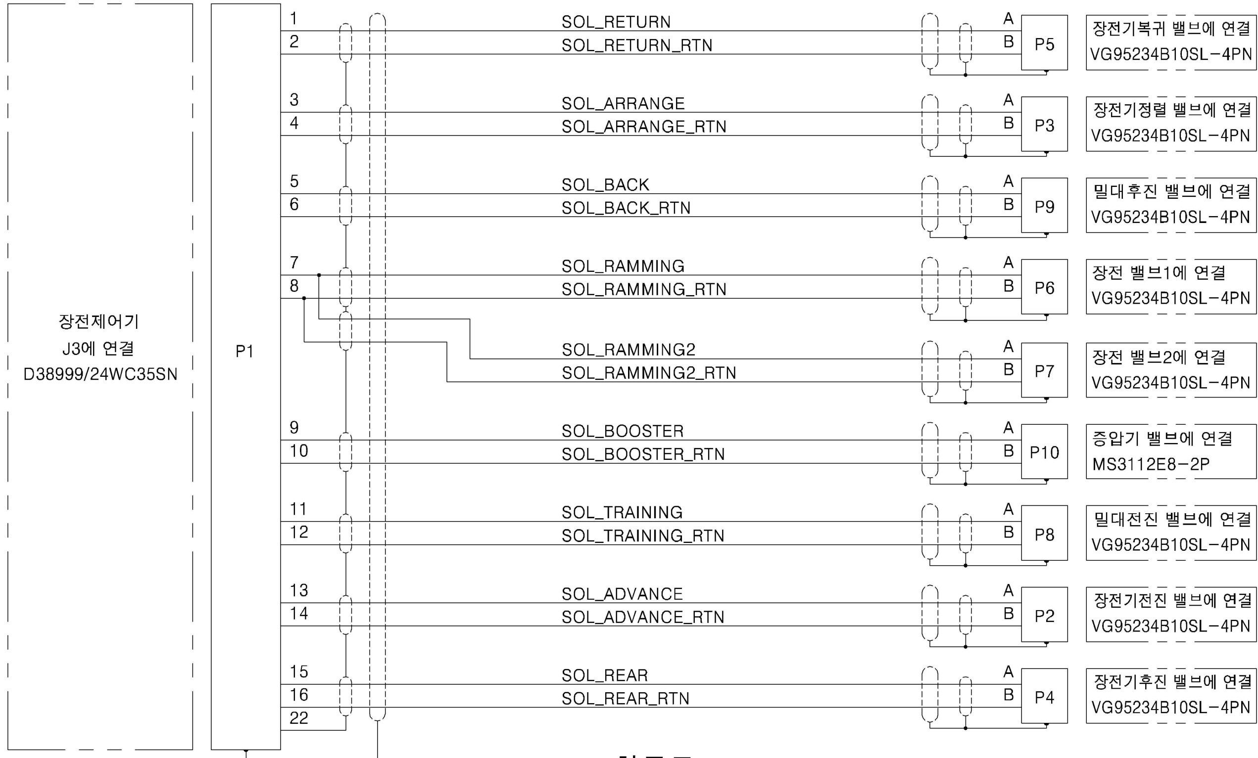
회로도
