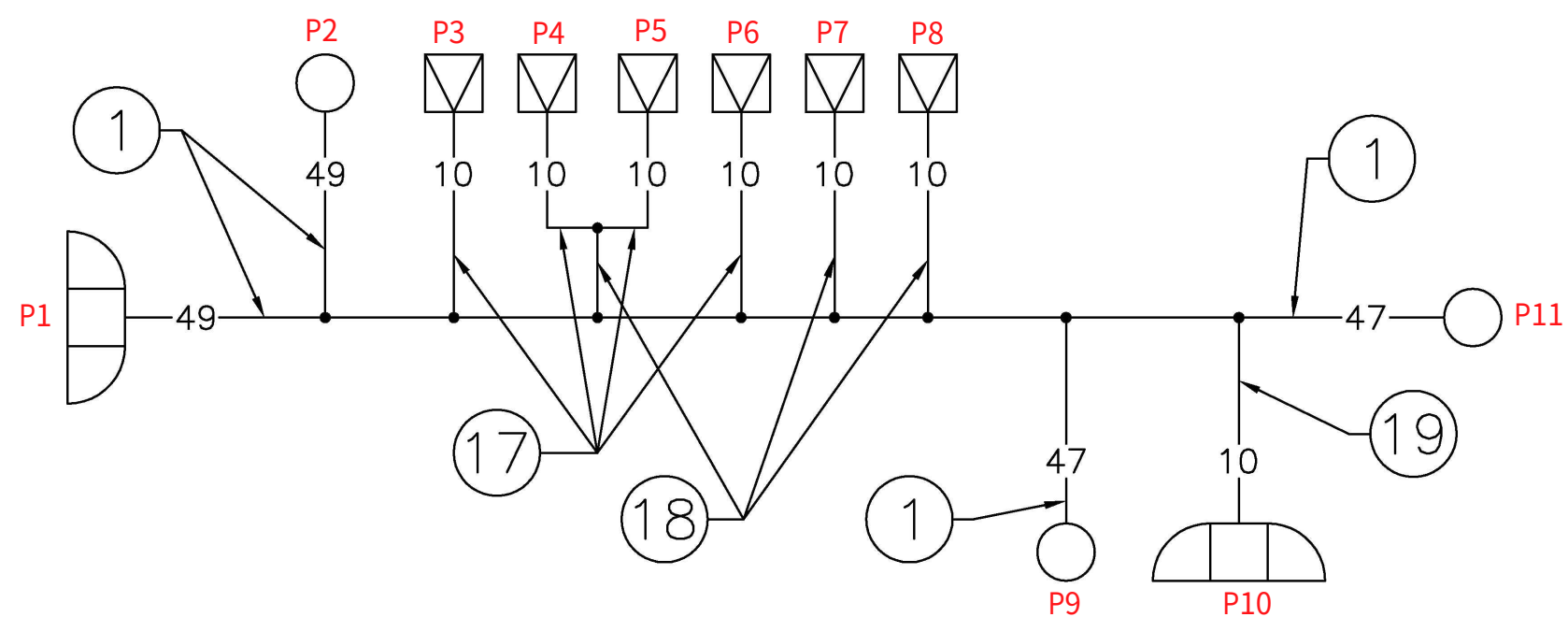
배선도
