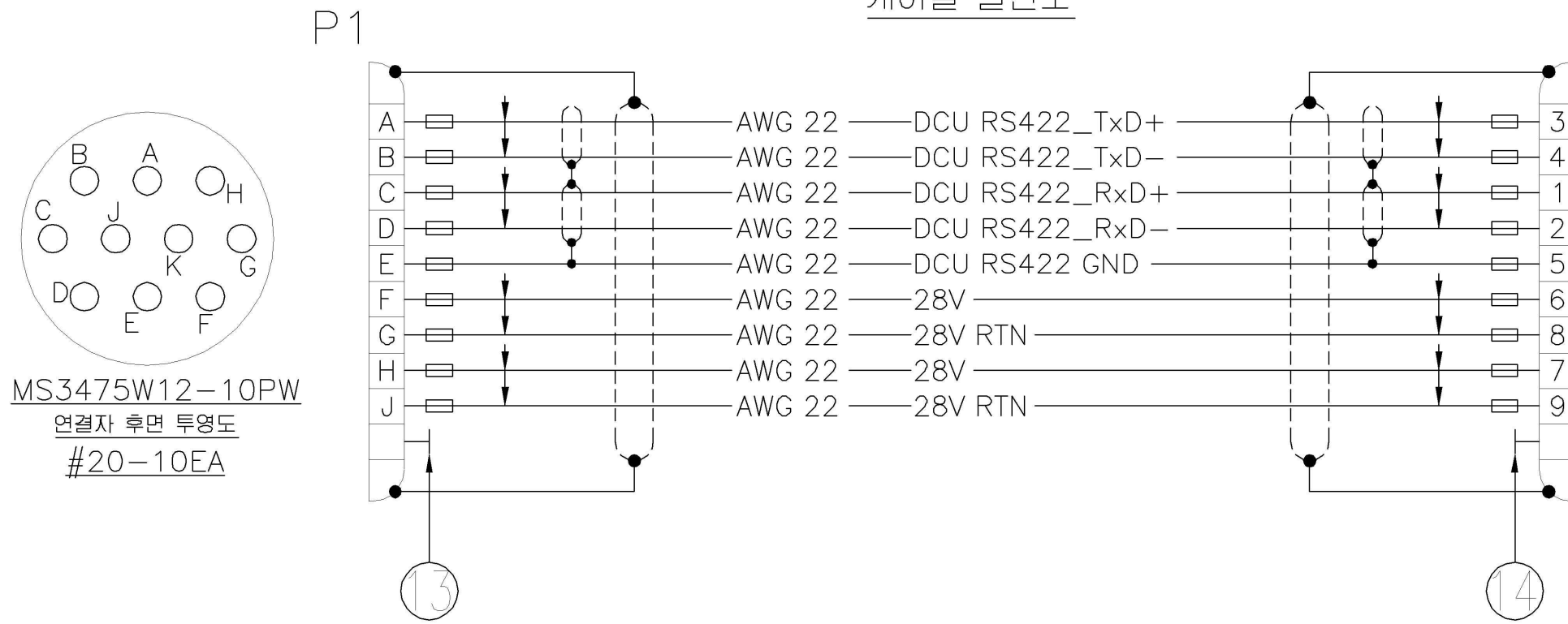
케이블 결선도
