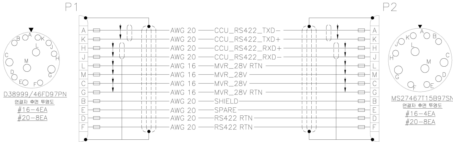
케이블 결선도
