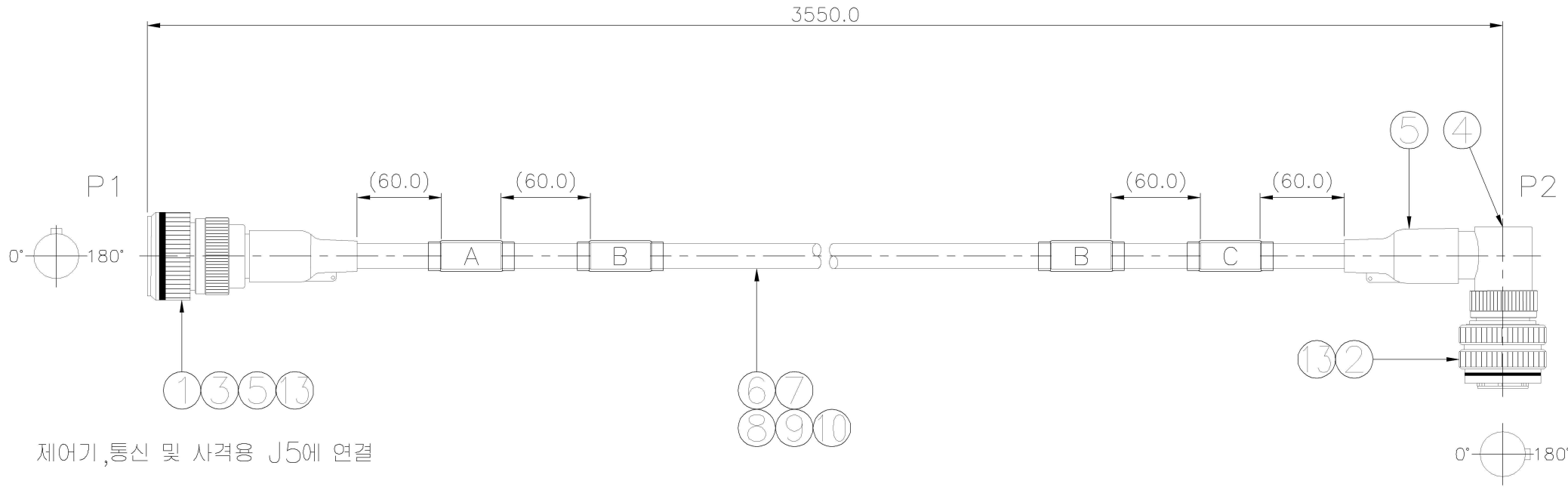
케이블 결선도
