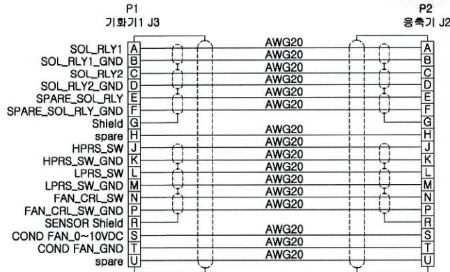
배선도
