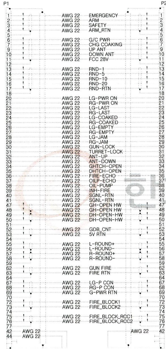
케이블 결선도
