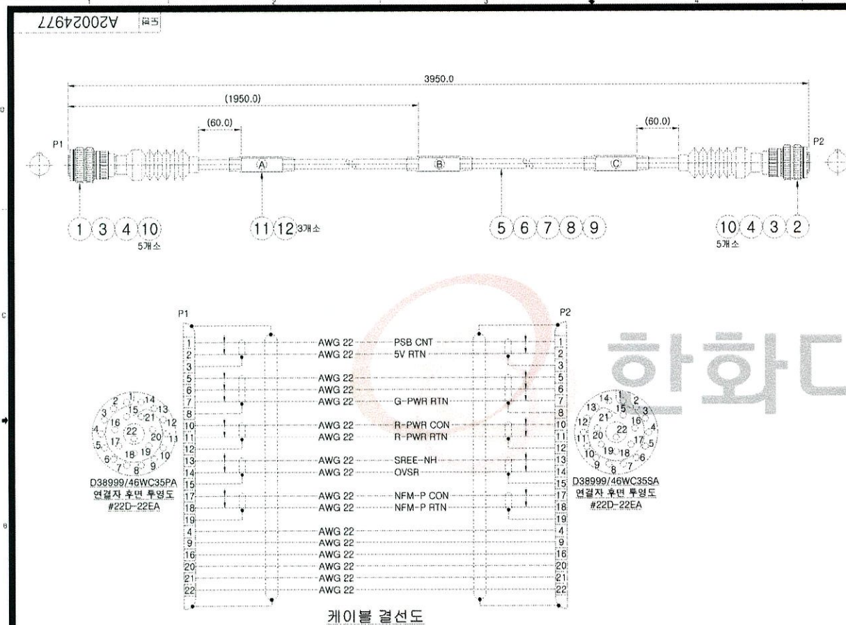
케이블 결선도
