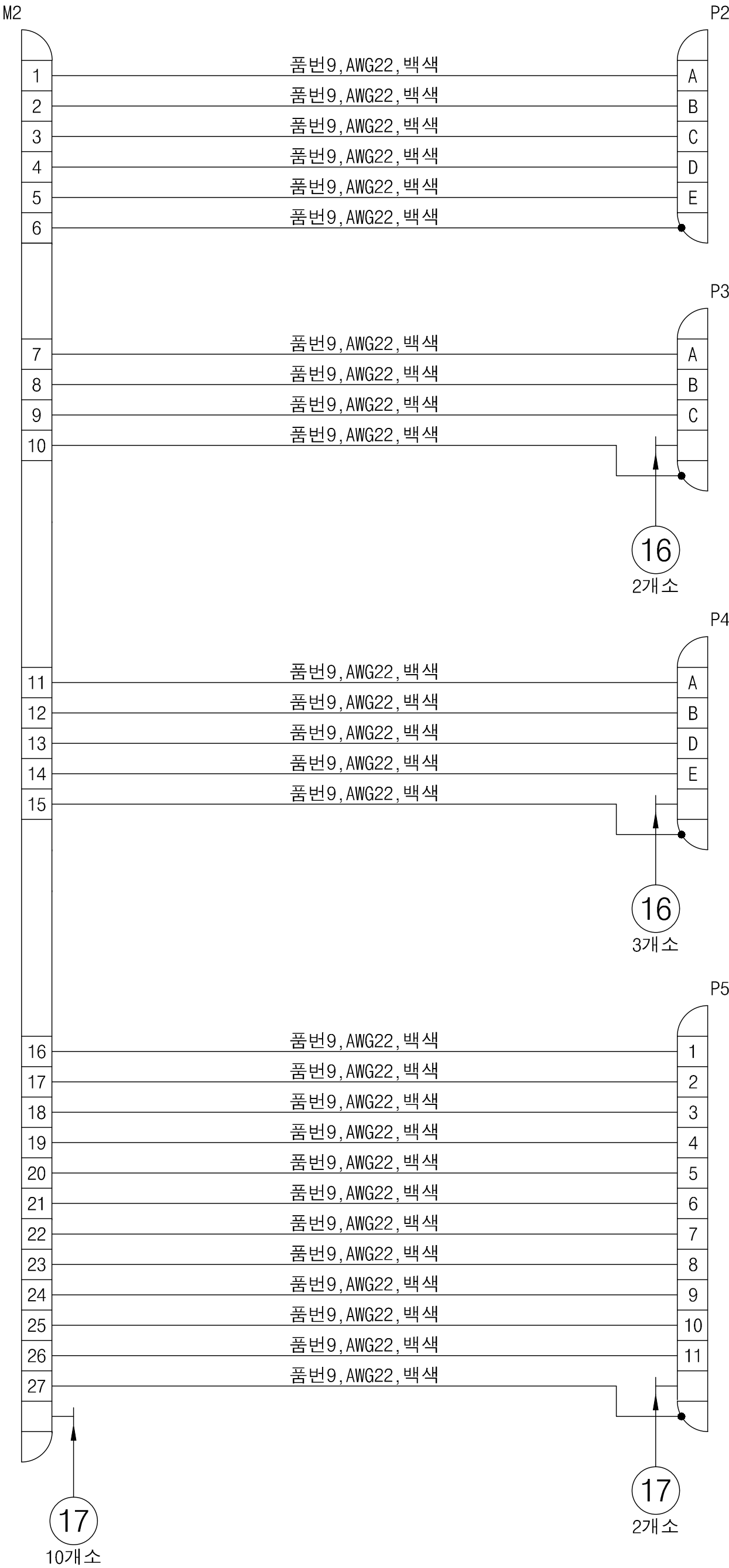
배선도
