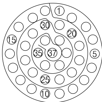
YH38999/46WD35SN 연결기 후면도 #22D-37EA
