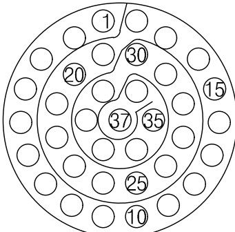
YH38999/46WD35PN 연결기 후면도 #22D-37EA
